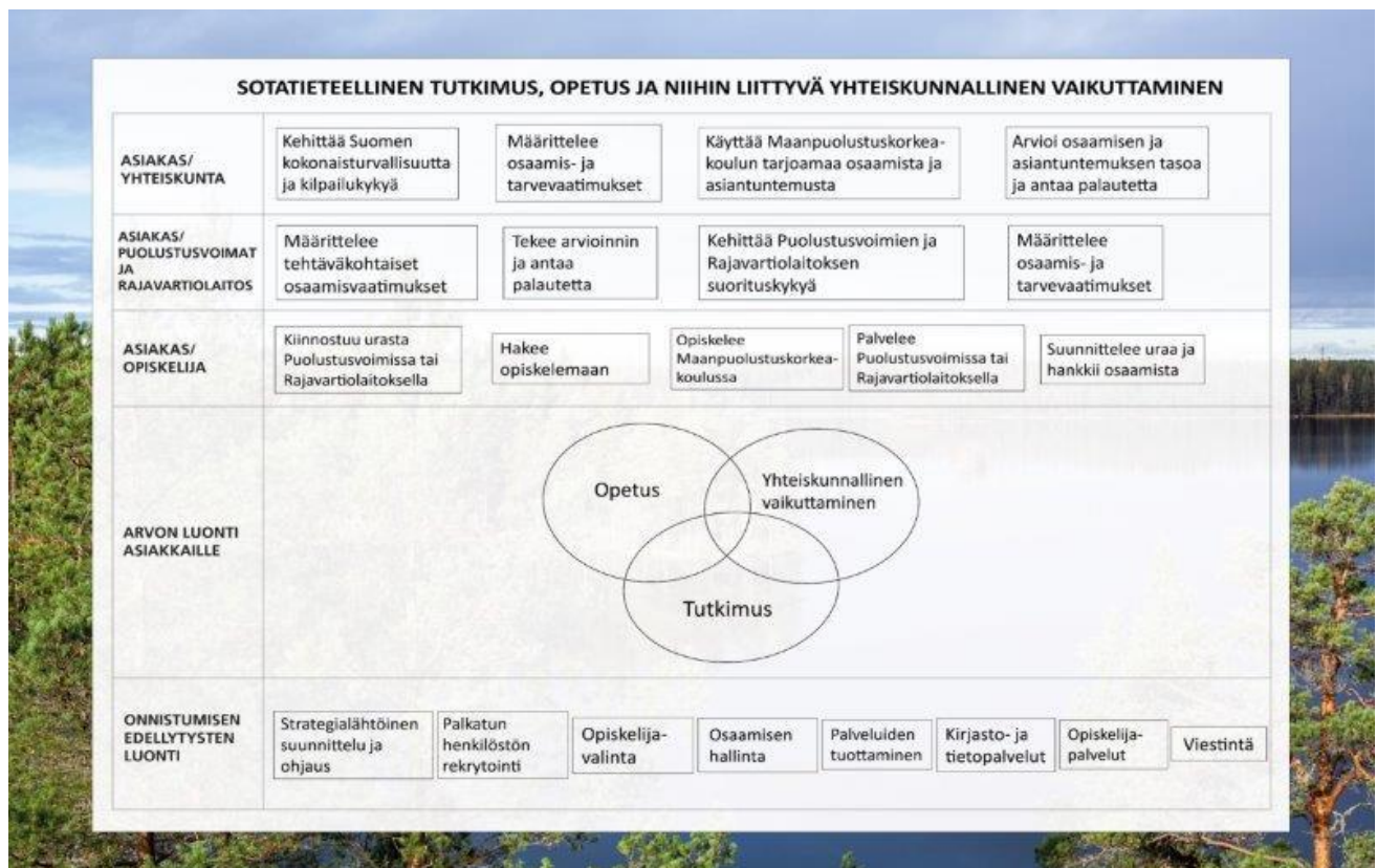
Kuva 3: Maanpuolustuskorkeakoulun prosessikartta
